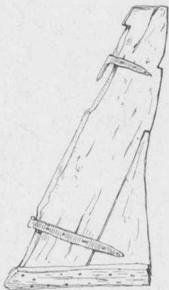
Roer van het turfschip, aanwezig in het Rijksmuseum te Amsterdam. ( 1 / 15 der ware grootte).
