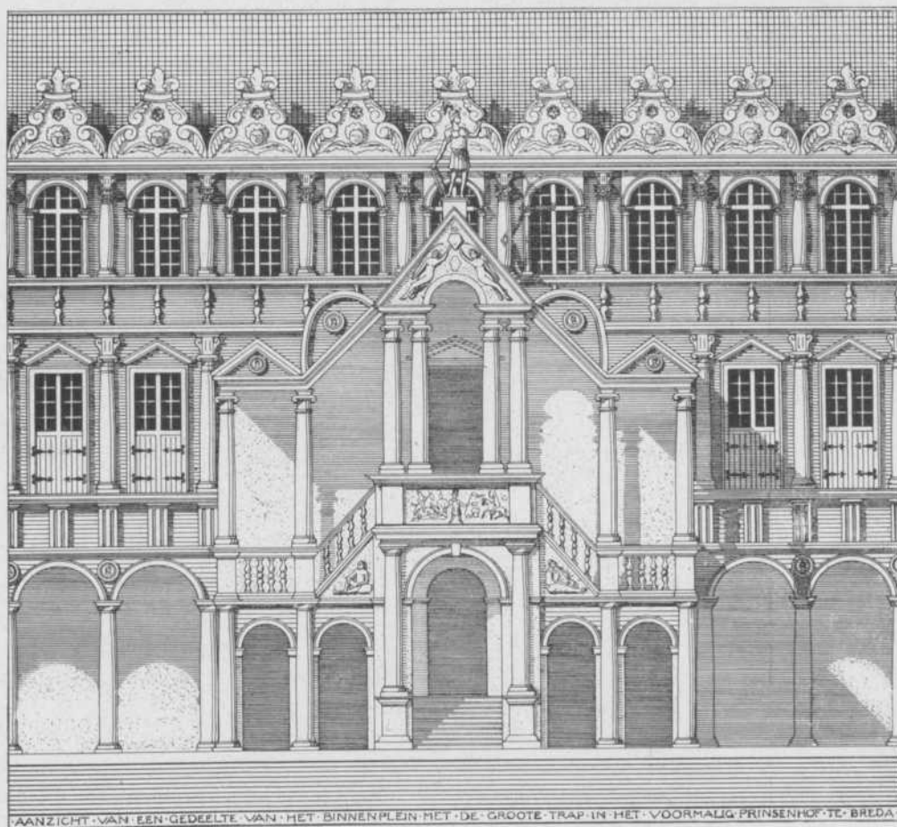
Groote trap op het binnenplein. Naar eene teekening in de Bibliotheek der Kon. Mil. Academie.
