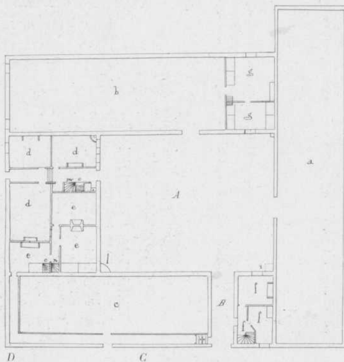
Plattegrond van Zijne Hoogheids stallen en Koetshuys, Kaatsbaan, Tuinierswoning en verder Logement te Breda. Naar een teekening in het Rijksarchief te 's Hertogenbosch.
